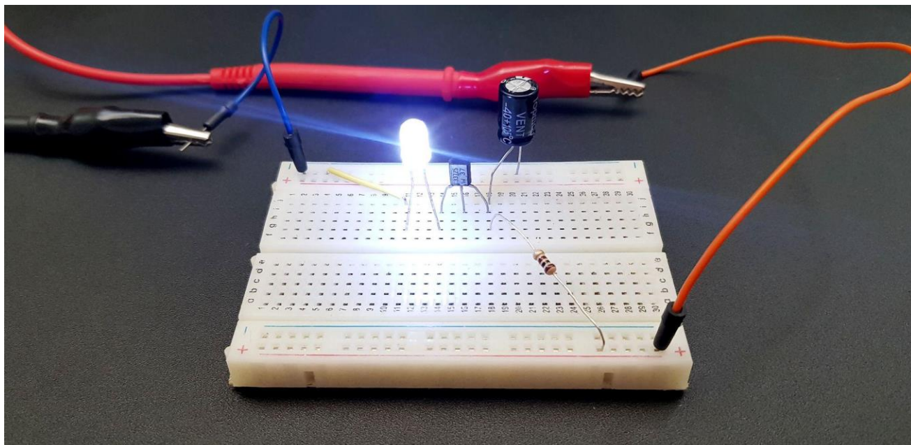
Figura 17 - Foto capturada no momento em que o capacitor descarrega e a corrente passa pelo transistor, acendendo o LED.
