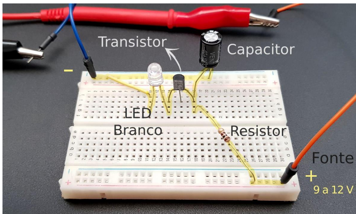
Figura 15 - Circuito LED blinker utilizado para o experimento. O realce amarelo representa o caminho percorrido pelos elétrons no circuito.
