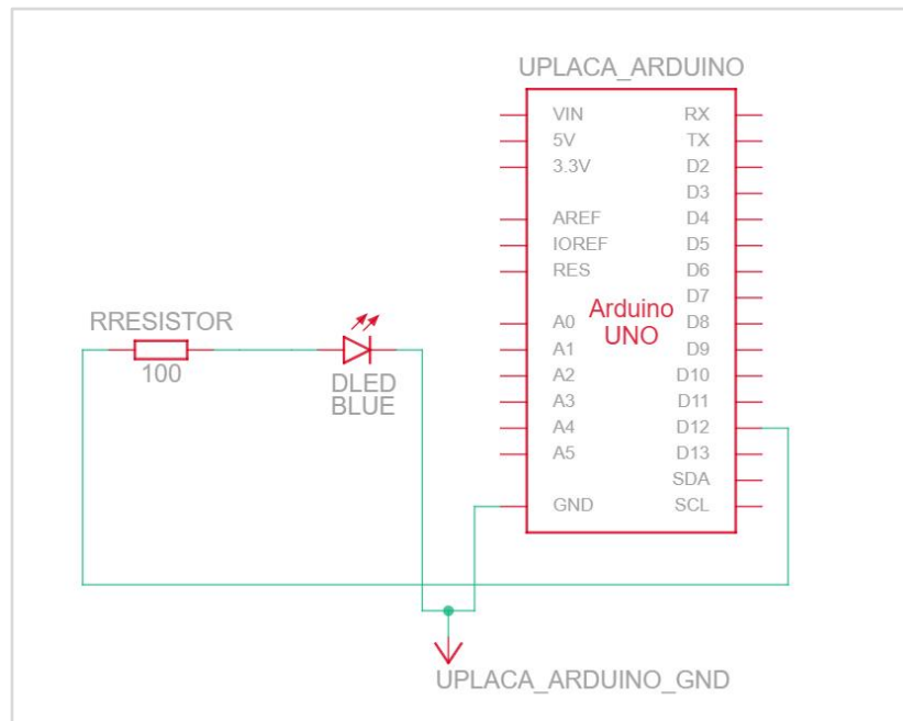
Figura 43 - Diagrama esquemático do circuito LED blinker para Arduino.
