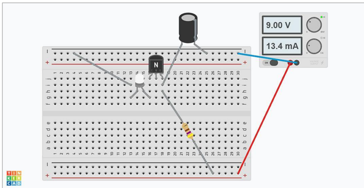
Figura 16 - Simulação do circuito LED blinker realizada na plataforma Tinkercad.
