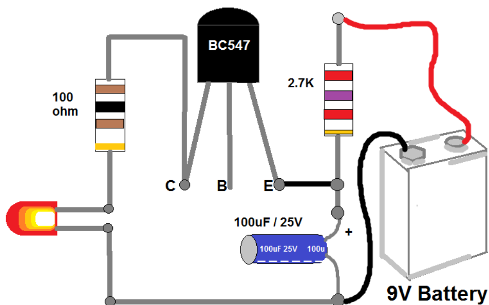
Figura 14 - Representação genérica de um circuito LED blinker .
