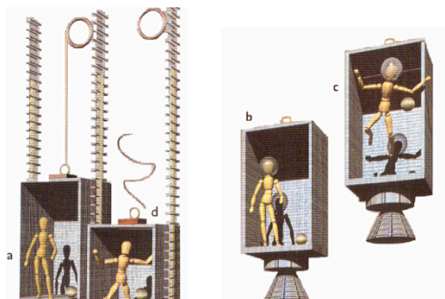
Figura 14. Princípio da equivalência (elevador x foguete).
